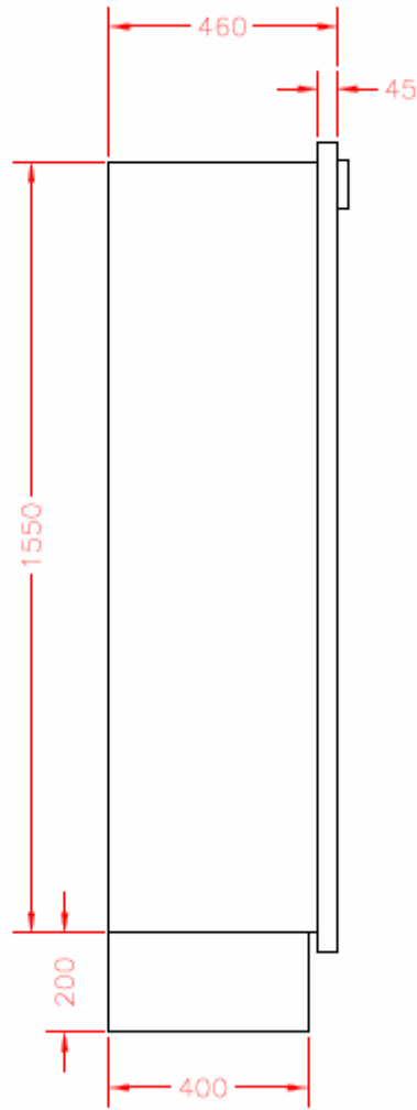
VISTA LATERAL
